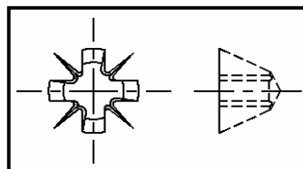
Pozi Recess
